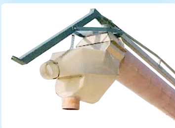
Séparateur d'eau et attache tracteur
