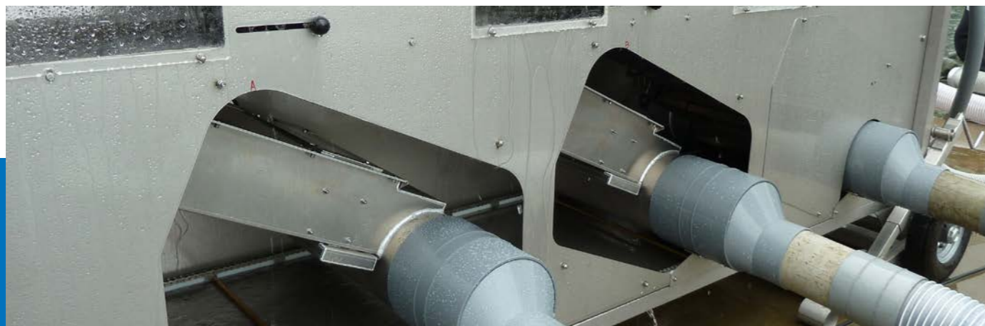
Los contadores Pescavision situados en el clasificador son de fácil acceso.
