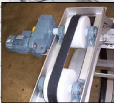
Entraînement du tambour par une courroie.
