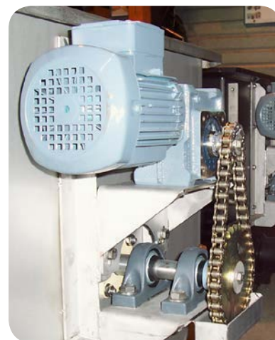
Entrainement du tambour par chaîne.
