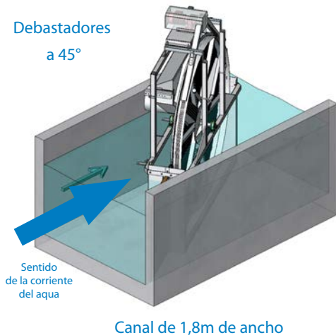
DEBASTADORES Ø2200 - Vista por el costado de llegada del agua
